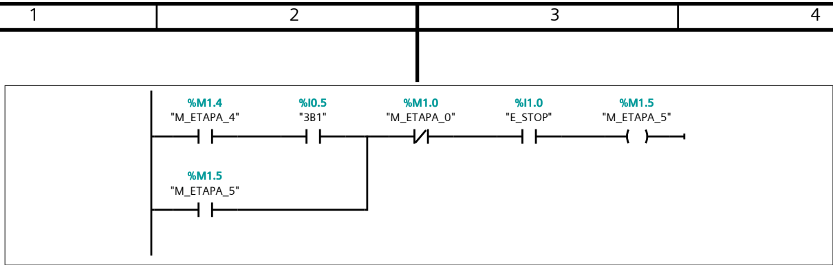
Network 10: Orden interna: Retraer Rotativo y Cilindro 2
