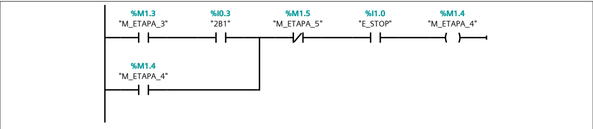
Network 9: Retorno simultáneo Rotativo y Cilindro 2
