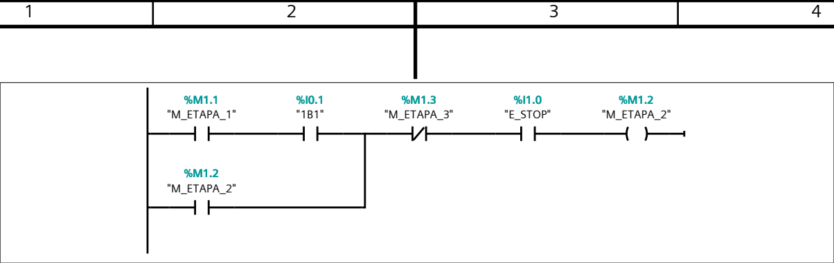
Network 7: Retorno simultáneo Rotativo y Cilindro 2
