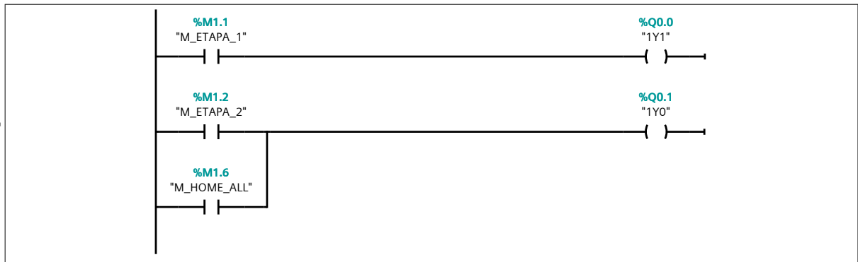
Network 12: Solenoide Giro Rotativo (Orientación 0° a 90°)
